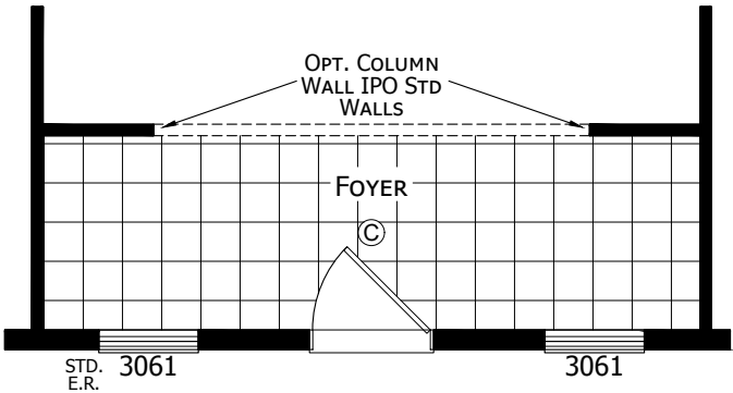
OPTIONAL FOYER
